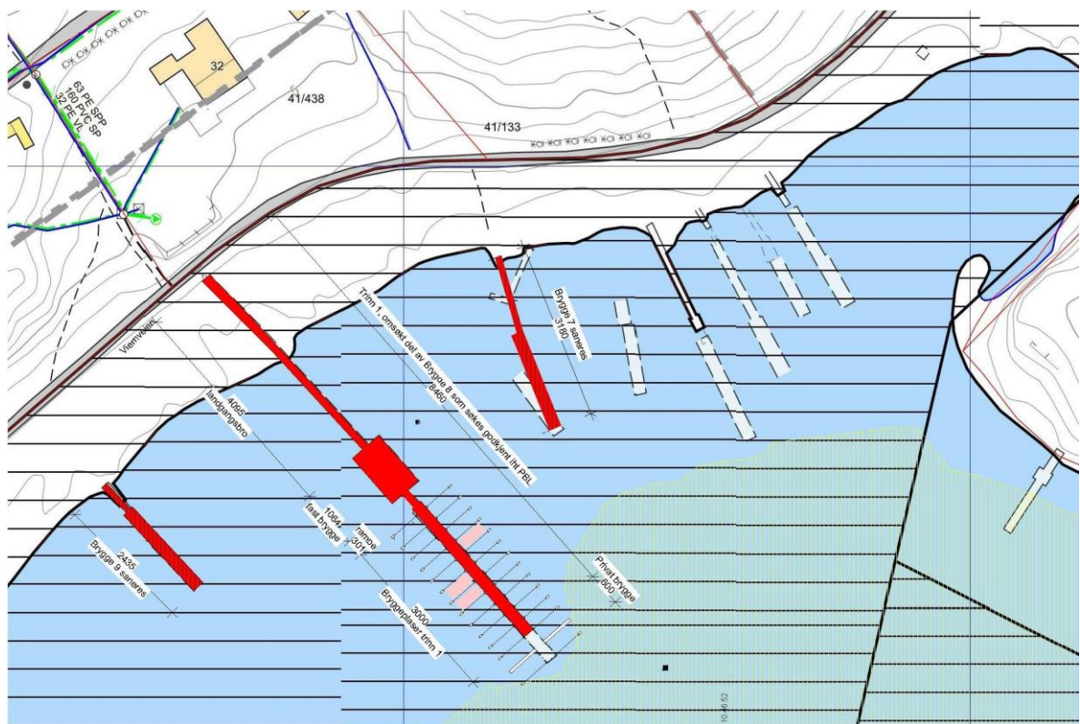
Figur 3. Plantegning av bryggeanlegget slik det er framstilt i Trinn 1 ovenfor. De to mindre bryggene på hver sin side av fellesbrygga som også er farget røde, skal rives i forbindelse med dette byggetrinnet. Målene er oppgitt i cm.
