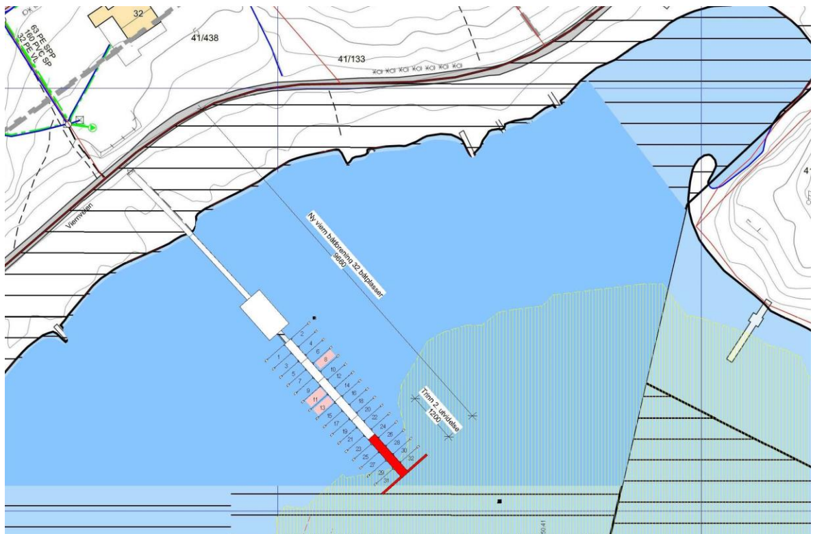
Figur 4. Plantegning av bryggeanlegget slik det er framstilt i Trinn 2 ovenfor. Her er alle de små bryggene fjernet. Målene er oppgitt i cm.
