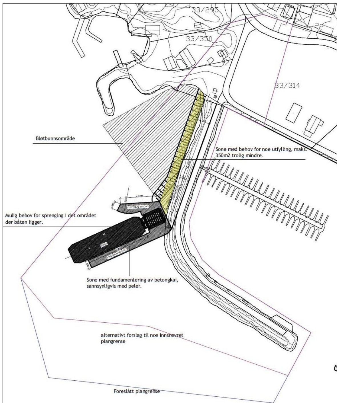
Figur 2a. Planskisse av det nye fergeleiet på Sandøya. Merk at ferge er tegnet inn i illustrasjonen.
