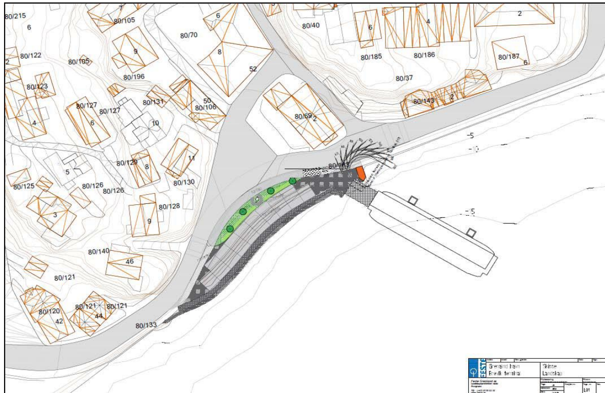
Figur 2b. Planskisse av det nye fergeleiet i Brevik sentrum. Omrisset av ferga er tegnet inn på planskissa.
